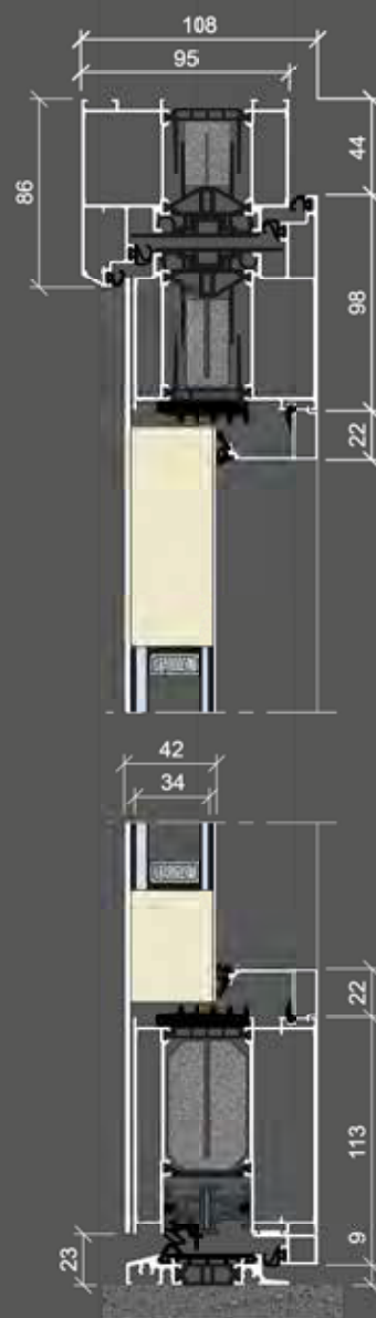
Ausführung mit schrägem Blendrahmen (optional): KÖSTER ADVANCE 108
